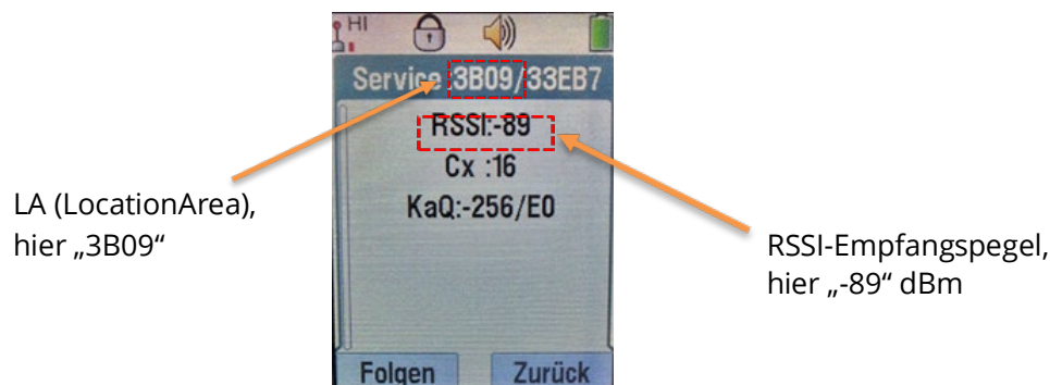
Abb.: Motorola HRT Display
